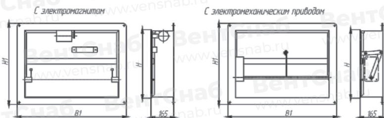
Стеновое исполнение
